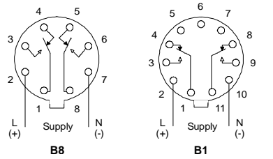
CONNECTION DIAGRAM DIAGRAMME DE CONNECTION SCHALTBILDANSCHLUSS
